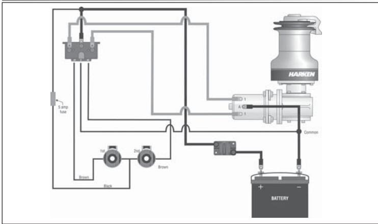
GB: WIRE SIZE CHART (distance in meters from battery to winch and back battery) • F: TABLEAU DE DIMENSION DES CABLES (distance en mètres de la batterie au winch et retour) • D: LEITER TABELLE (Länge von Batterie zur Winch und zurück zur Batterie) • I: Tabella dimensione cavi (Distanza in metri dalla batteria al winch e ritorno alla batteria) • E: TABLA TAMAÑO CABLES (distancia en metros desde la Batería al winche y a la Batería posterior)
